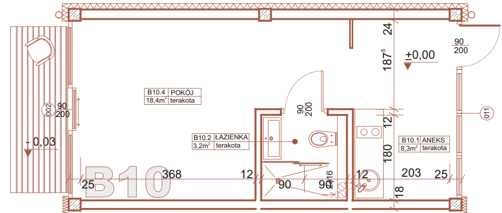
RZUT POZIOMY
